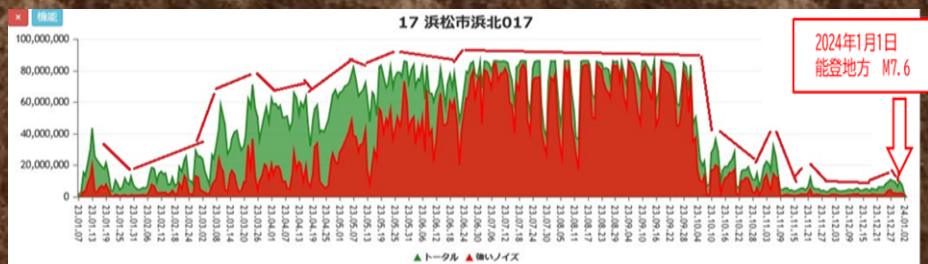
2024年（令和6年）1月1日能登地震M7.6の前兆データ
